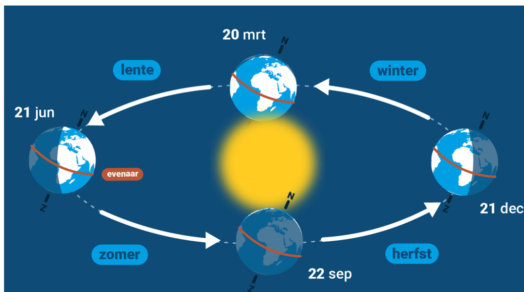
De astronomische seizoenen. Bron: Weerplaza.com.
